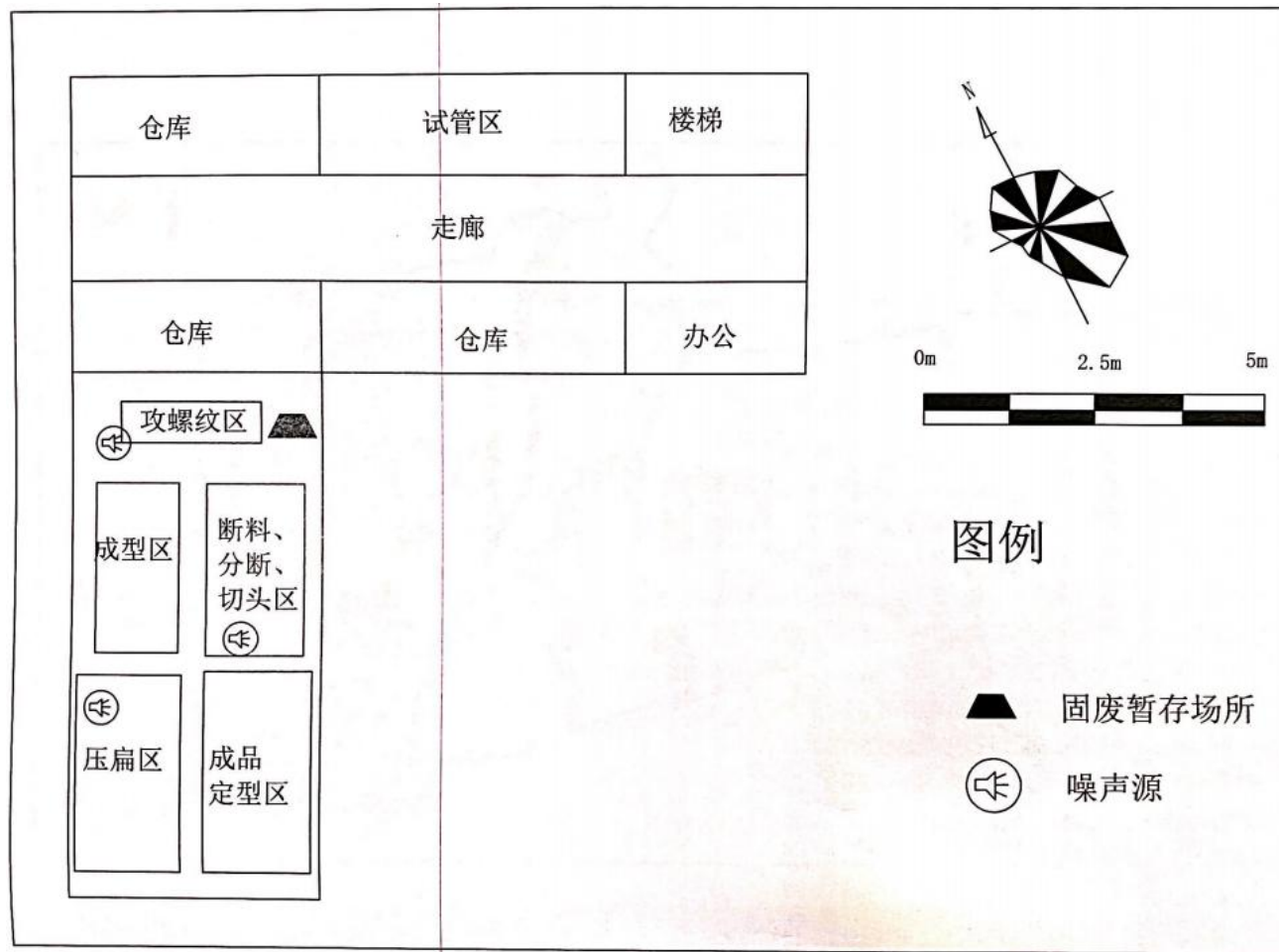
附图 3 项目车间平面布置图
