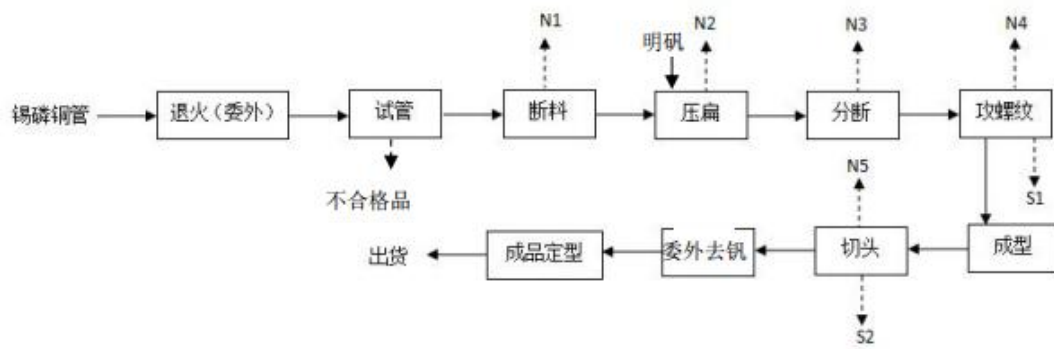
图 3.5-1 项目生产工艺流程图
